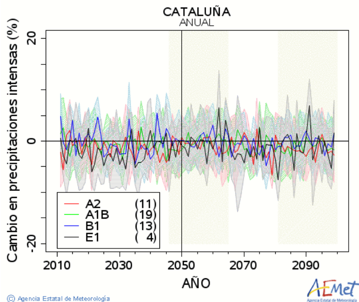
Figura 16: Proyecciones de cambio en las precipitaciones intensas para Cataluña, bajo los escenarios A2, A1B, B1 y E1.
