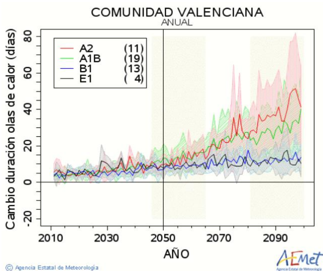
Figura 8: Proyecciones de cambio en la duración de las olas de calor para la Comunidad Valenciana, bajo los escenarios A2, A1B, B1 y E1.
