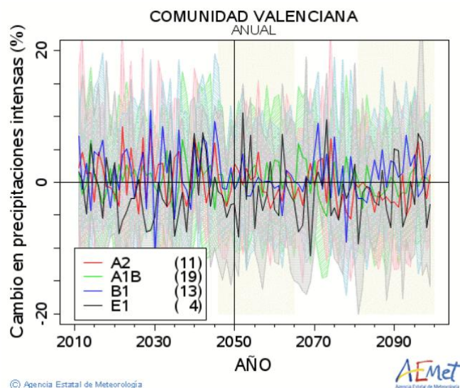
Figura 10: Proyecciones de cambio en las precipitaciones intensas para la Comunidad Valenciana, bajo los escenarios A2, A1B, B1 y E1.
