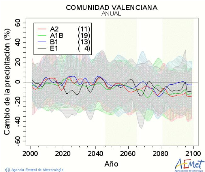
Figura 7: Proyecciones de variación porcentual de la precipitación media anual para la Comunidad Valenciana, bajo los escenarios A2, A1B, B1 y E1. Fuente: AEMET 36 .
